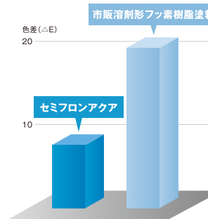
■セミフロンアクア汚染性データ (東京6ヶ月)
